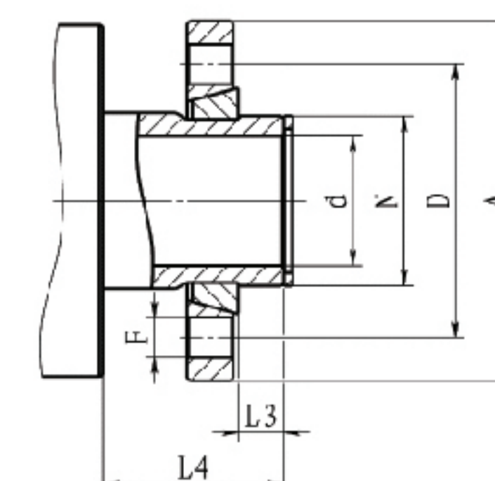
HS-X 双通/旋转式内管 DUAL FLOW ROTARY INTERNAL PIPE
