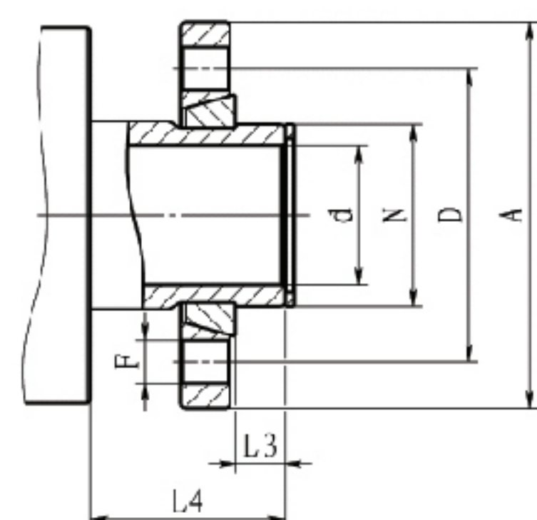
HD 单通 MONO FLOW
